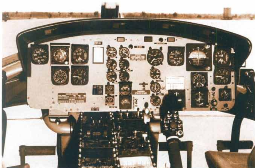
◀ Panel sterowania śmigłowca UH-1D / Bell
