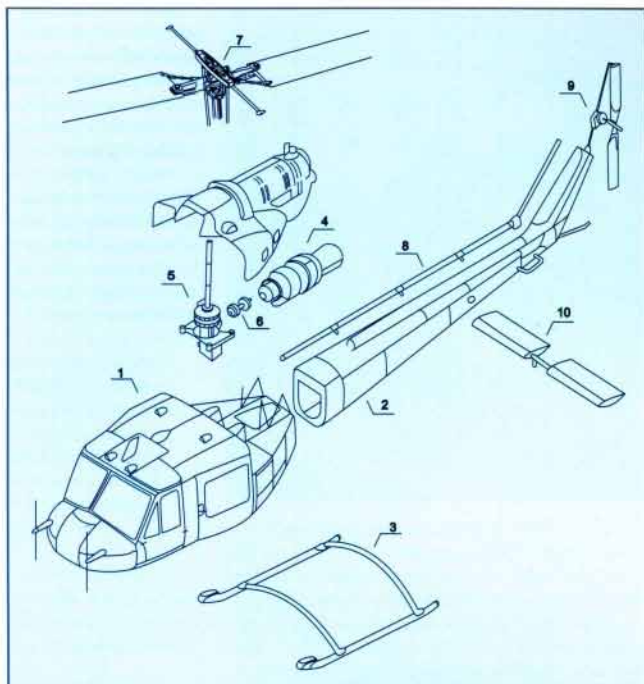
▲ Konstrukcja śmigłowca UH-1 — najważniejsze komponenty (główne sekcje konstrukcji śmigłowca UH-1B) / rys. Filip Kozarski
